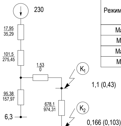
Схема замещения
